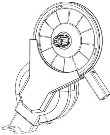
FUEGO 1.0 bike trainer main unit
