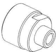
Adapter A – pour écrou de cassette à dégagement rapide
